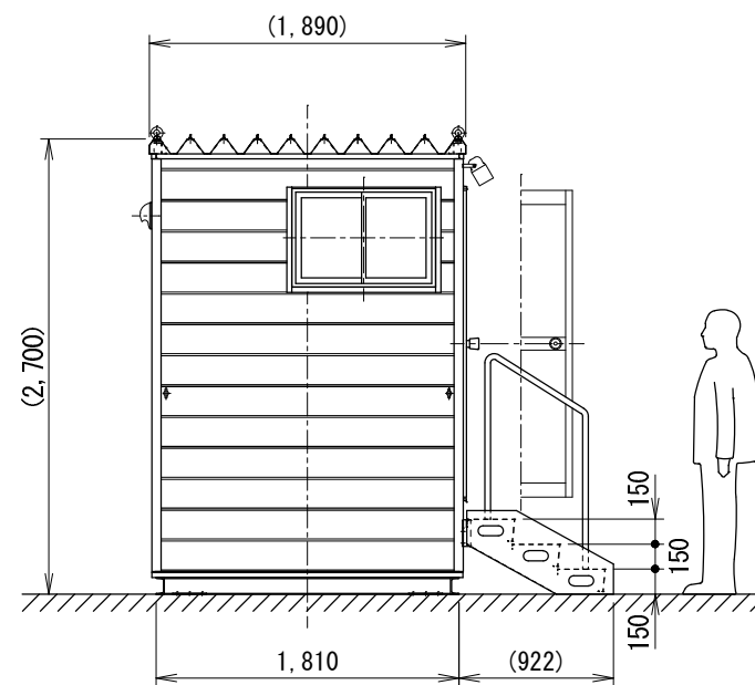
左側面図
