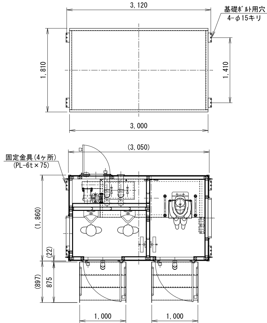
基礎* 用穴位置図
