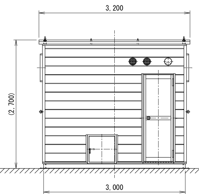
背面図
