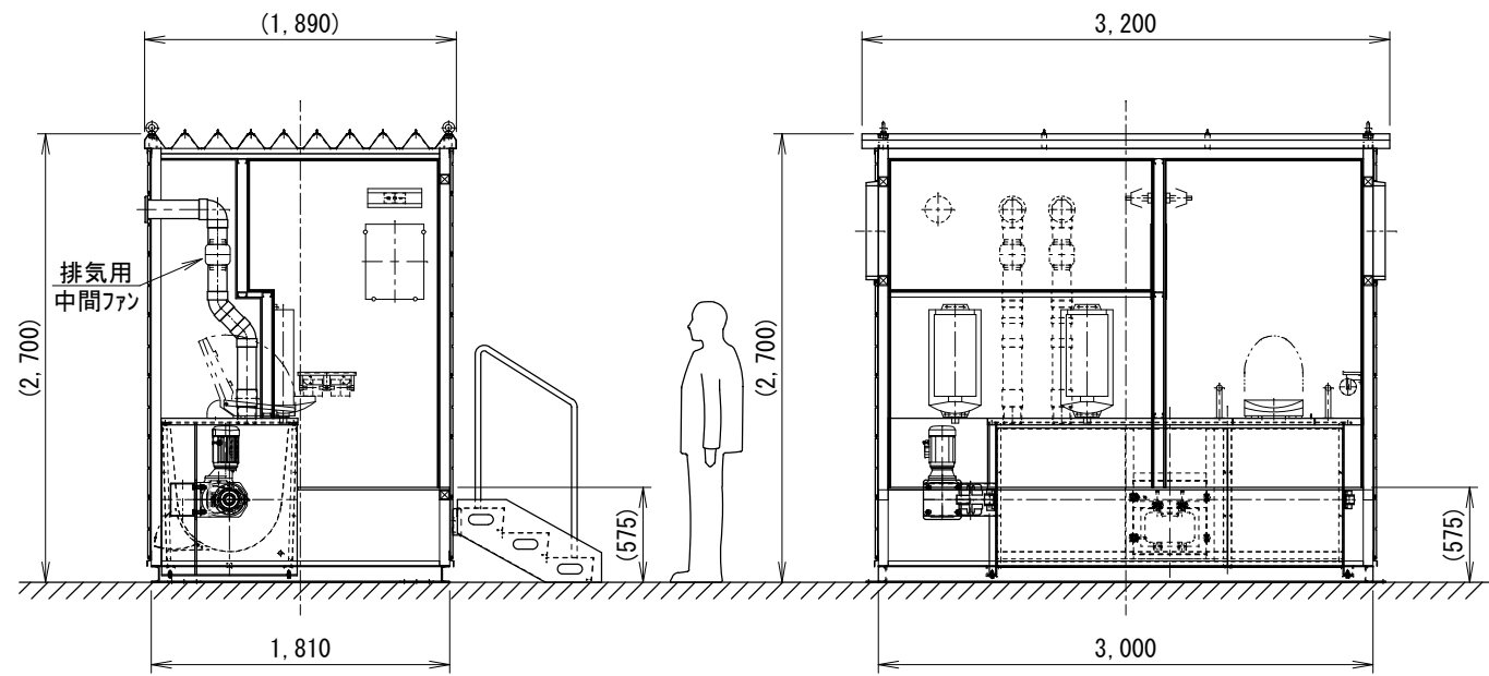
内観図
