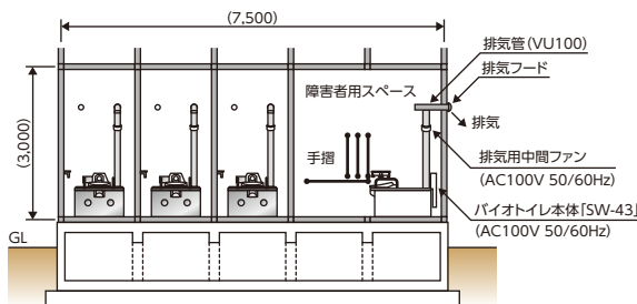
公衆トイレ参考配置断面図
