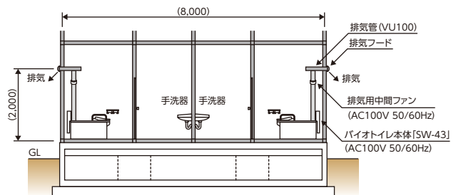
公衆トイレ参考配置断面図
