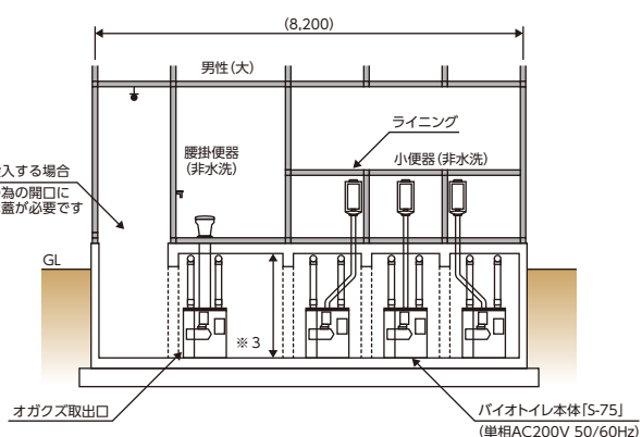
公衆トイレ参考配置断面図
