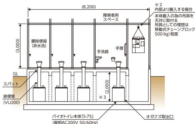
公衆トイレ参考配置断面図
