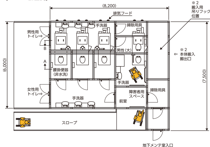
公衆トイレ参考配置平面図
