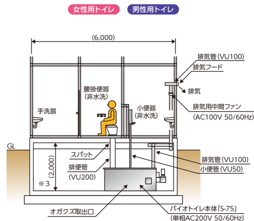
公衆トイレ参考配置断面図
